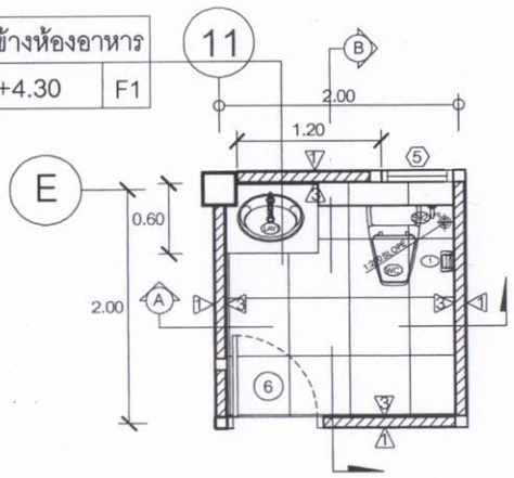
TL-3 AD- แบบขยายห้องน้ำ 3
